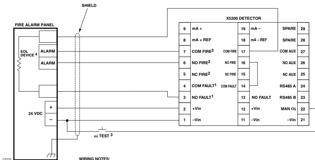
Figura 7 – Opção de Cabeamento Ex d
