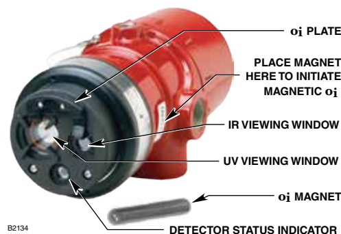
Figura 2 – Vista Frontal do X5200
