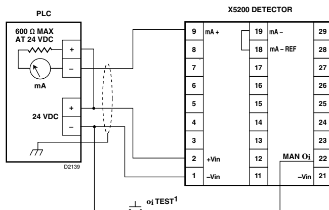
Figura 10 – Detector X5200 Instalado para Saída de Corrente de 0 a 20 mA Não Isolada (Declínio)
