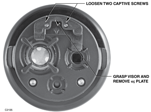
Figura 18 — Remoção da Placa O i
