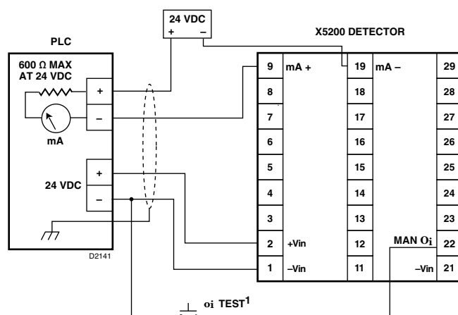
Figura 12 — Detector X5200 Instalado para Saída de Corrente de 0 a 20 mA isolada (Declínio)
