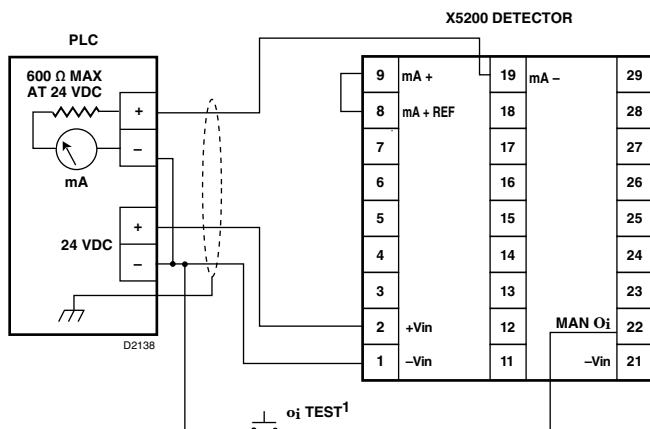
Figura 9 – Detector X5200 Instalado para Saída de Corrente de 0 a 20 mA Não Isolada (Fonte)
