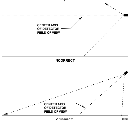
Figura 1 – Orientação do detector em relação ao horizonte
