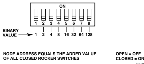
Figura 17 – Chaves de Endereço para X5200
