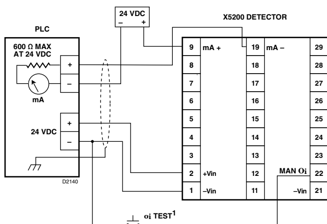
Figura 11— Detector X5200 Instalado para Saída de Corrente de 0 a 20 mA isolada (Fonte)
