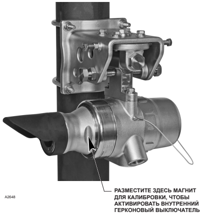
Рис. 2 — Расположение внутреннего магнитного выключателя на модуле приемника
