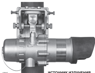
Рис. 3 — Идентификация модулей источника излучения и приемника
