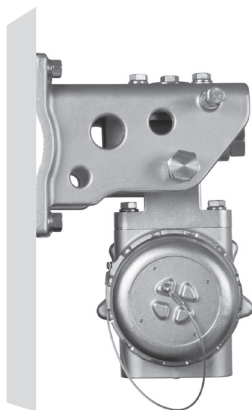
Рис. 10 — Газоанализатор LS2000, установленный на плоскую поверхность (Расстояние между отверстиями монтажной пластины см. в пункте «Габаритные размеры» раздела «Технические характеристики».)
