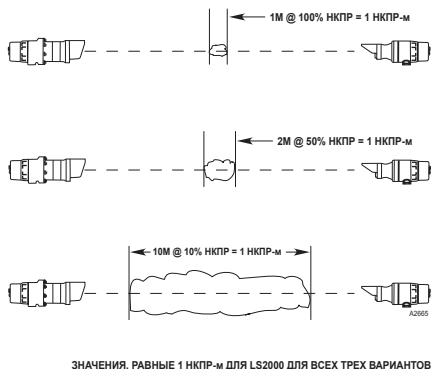
Рис. 1 — Отклик газоанализатора при обнаружении трех газовых облаков различного размера и концентрации
