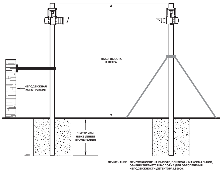
Рис. 8 — Пример распорки вертикальных опор для повышения надежности монтажа LS2000
