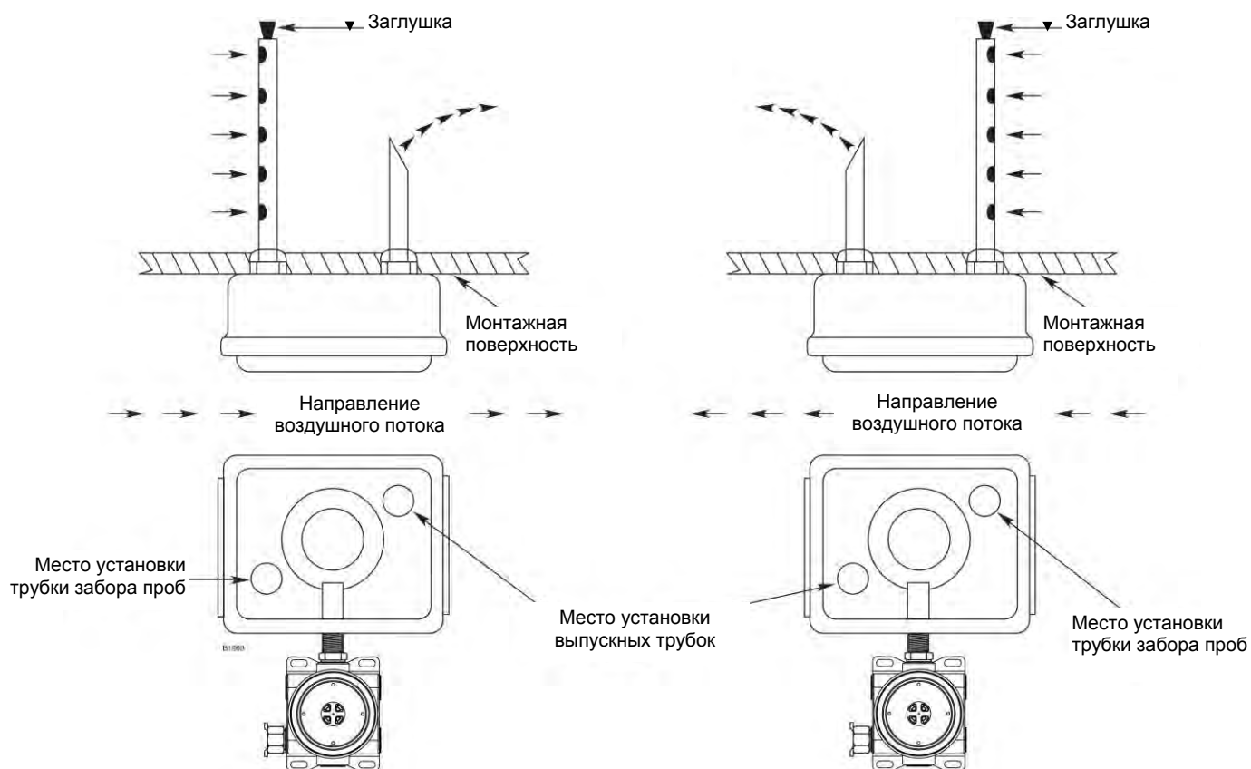
Рис. 3. Размещение и направленность трубок.
