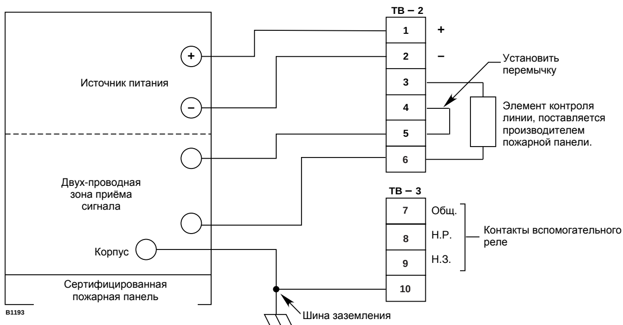
Рис. 5. . Схема подключения единичного извещателя
