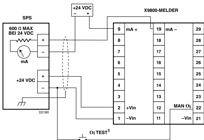
Abbildung 12 – X9800-Melderverdrahtung für isolierten 0-20-mA-Stromausgang (Sourcing)
