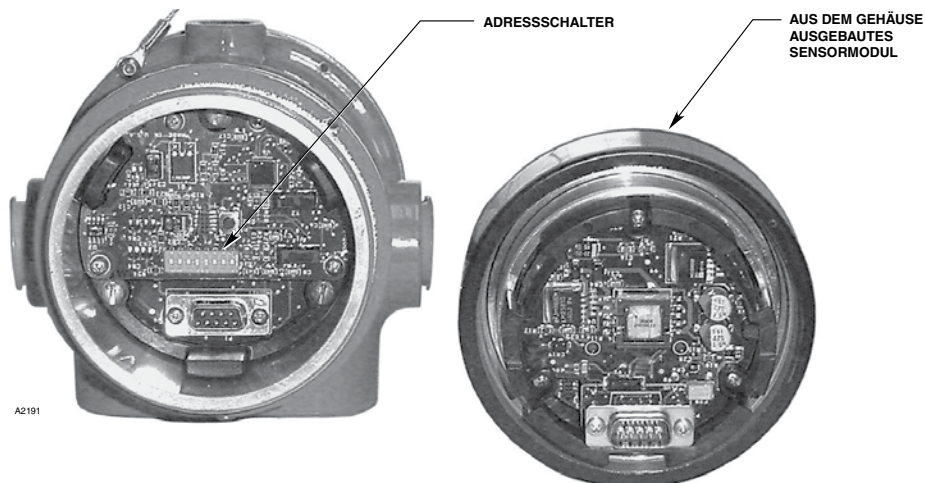
Abbildung 17 – Lage der Adressschalter
