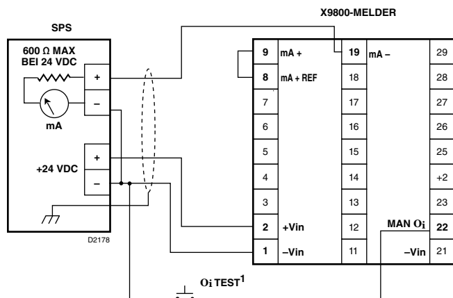
Abbildung 10 – X9800-Melderverdrahtung für nicht isolierten 0-20-mA-Stromausgang (Sourcing)
