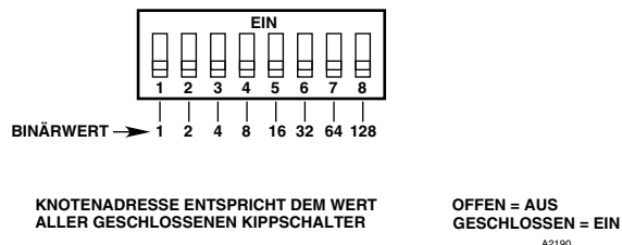
Abbildung 18 – Adressschalter für X9800
