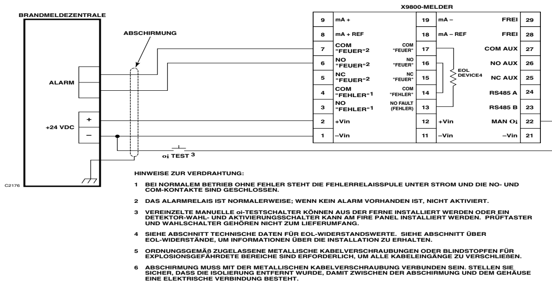
Abbildung 7 – Ex d-Verdrahtungsoption
