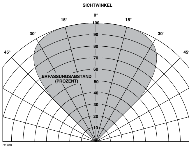
Abbildung 20 – Meldersichtkegel
