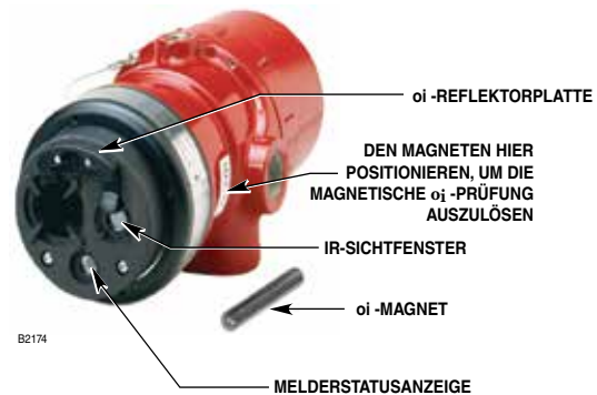
Abbildung 2 – Vorderansicht des X9800
