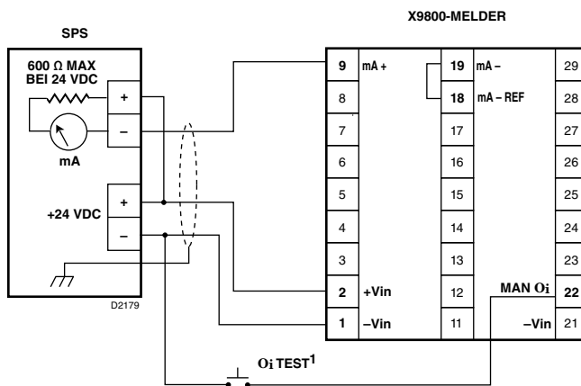
Abbildung 11 – X9800-Melderverdrahtung für nicht isolierten 0-20-mA-Stromausgang (Sinking)
