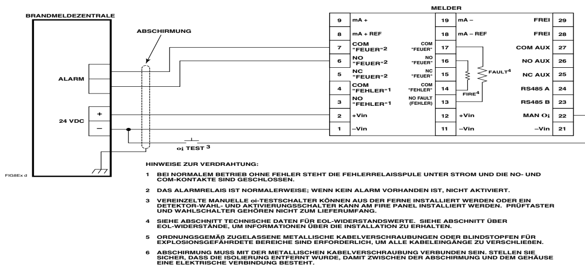
Abbildung 8 – Ex e-Verdrahtungsoption
