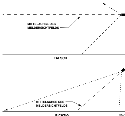
Abbildung 1 – Melderorientierung bezüglich des Horizonts
