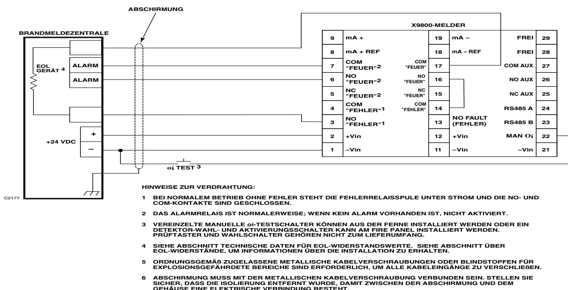
Abbildung 9 – Ex f-Verdrahtungsoption
