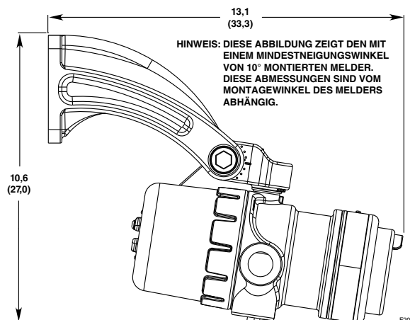
Abbildung 3 – Q9033 Montagearm ohne Abmessungen der Manschettenbaugruppe in Zoll (cm) (Angaben zur korrekten Melderorientierung siehe Abbildung 1.)
