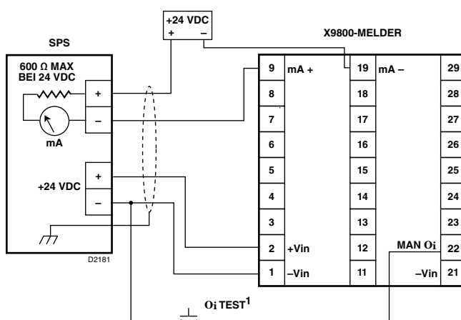
Abbildung 13 – X9800-Melderverdrahtung für isolierten 0-20-mA-Stromausgang (Sinking)
