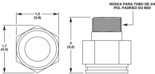
Figura 1—Dimensões do sensor em polegadas (centímetros)
